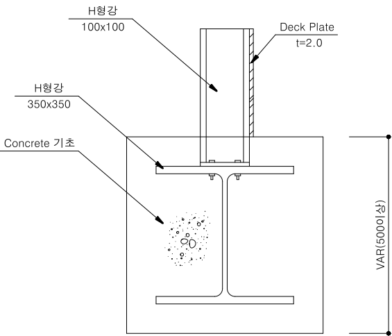
단 면 F-F
