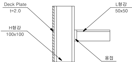
단 면 D-D
